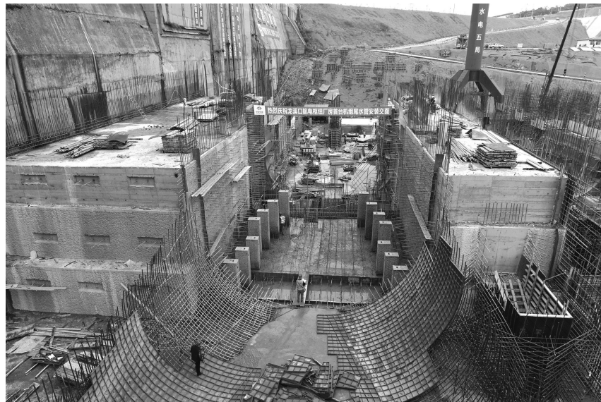
首台机组尾水管安装现场 受访单位供图
